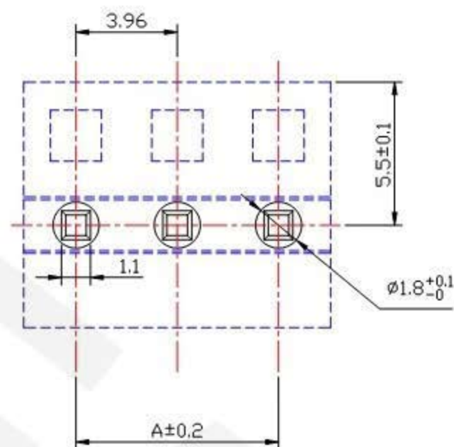
P.C.B LAYOUT
