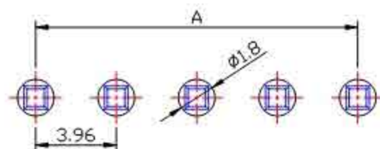
P.C.B LAYOUT
