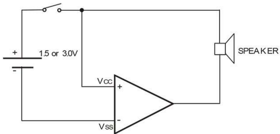
Рисунок 1. Схема включения BT8028C с использованием динамика
