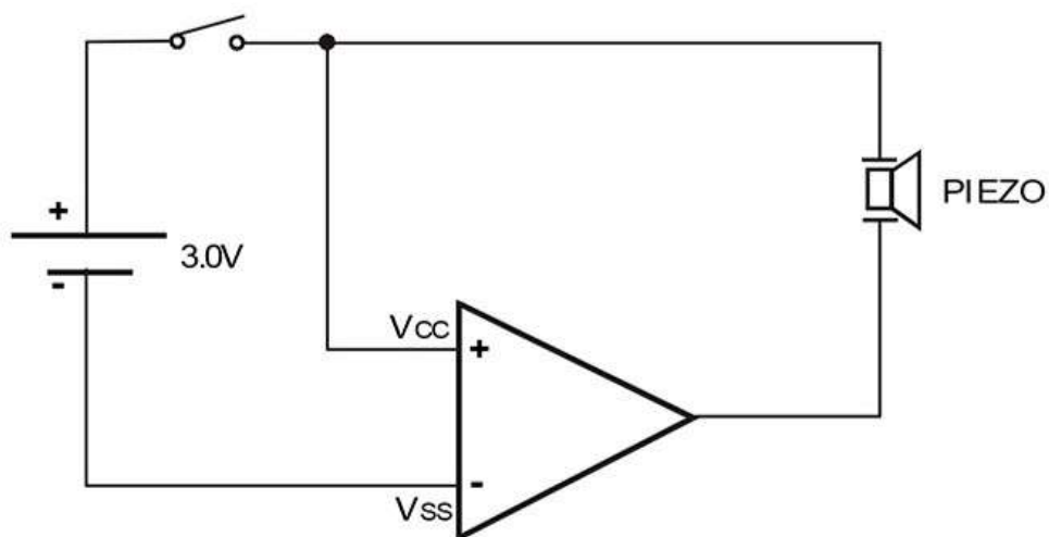
Рисунок 3. Схема включения BT8028C (прямая схема включения, пьезотип)
